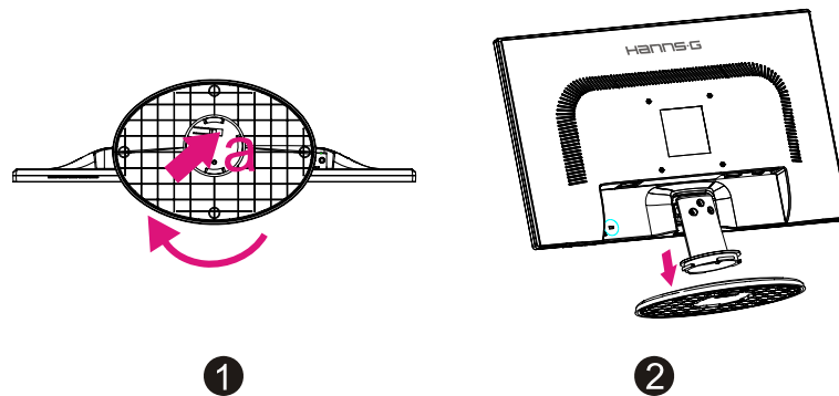
Instalação e remoção da base
