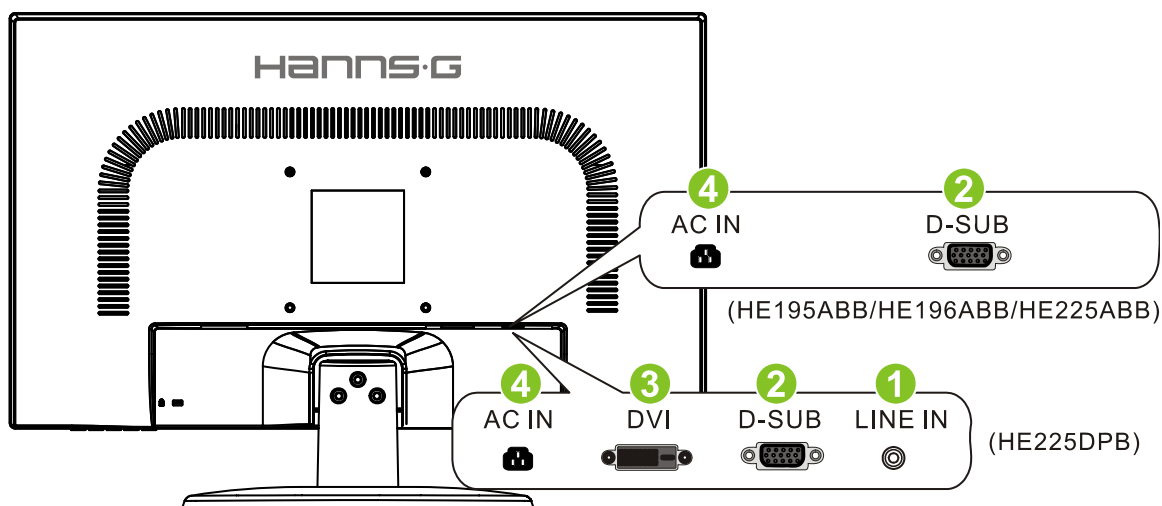
Figura 2. Ligação ao pc
