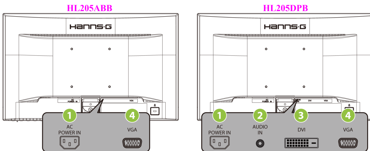
图二. 连接到 PC
