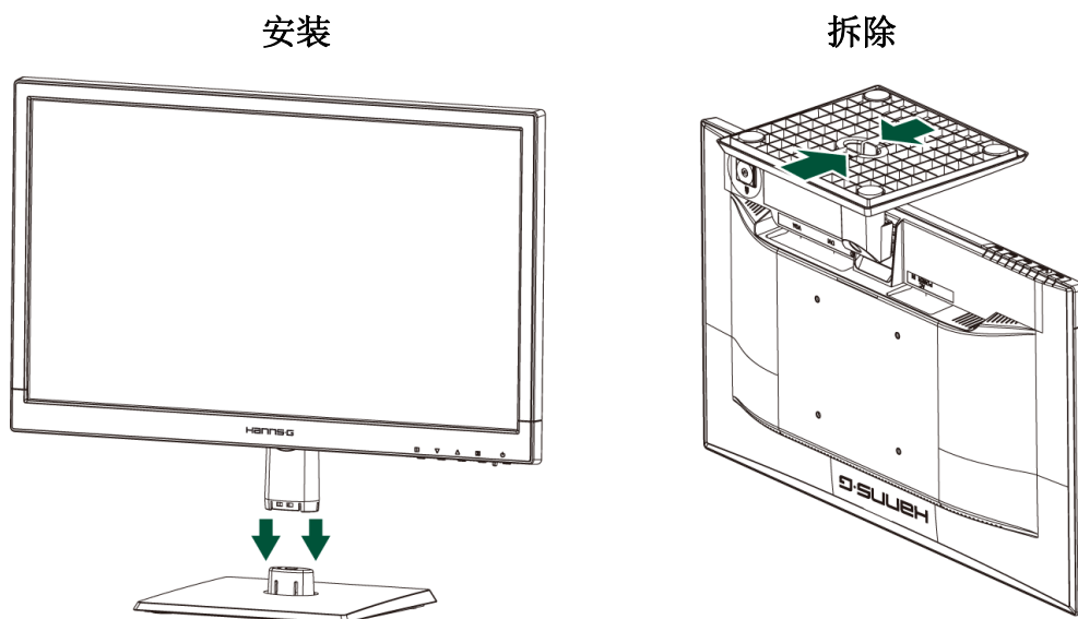
图一. 安装和拆除底座
