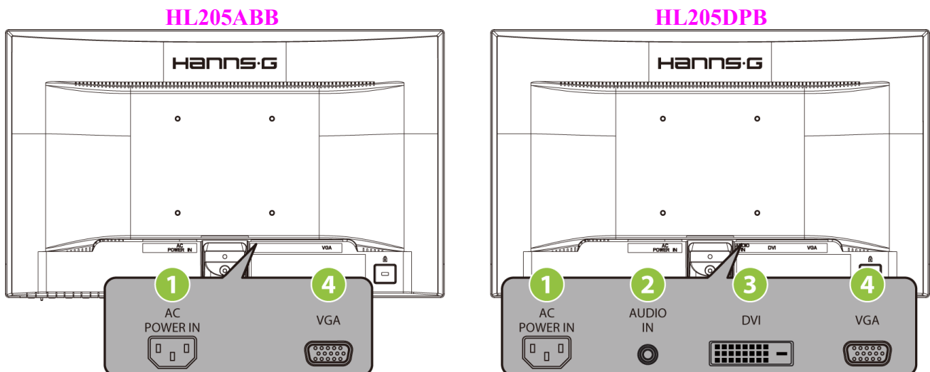
Bild 2. Koppla kablarna
