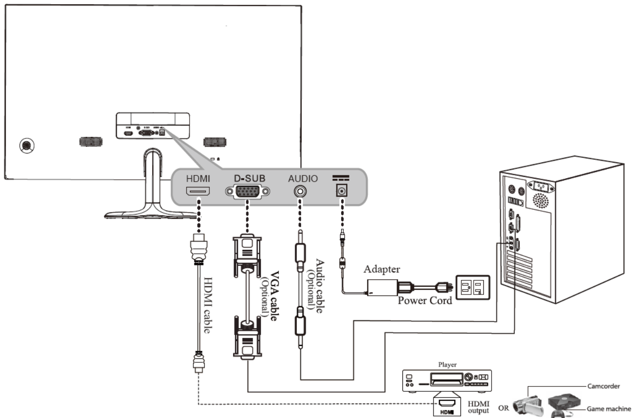
Figura 2. Conexión a un PC
