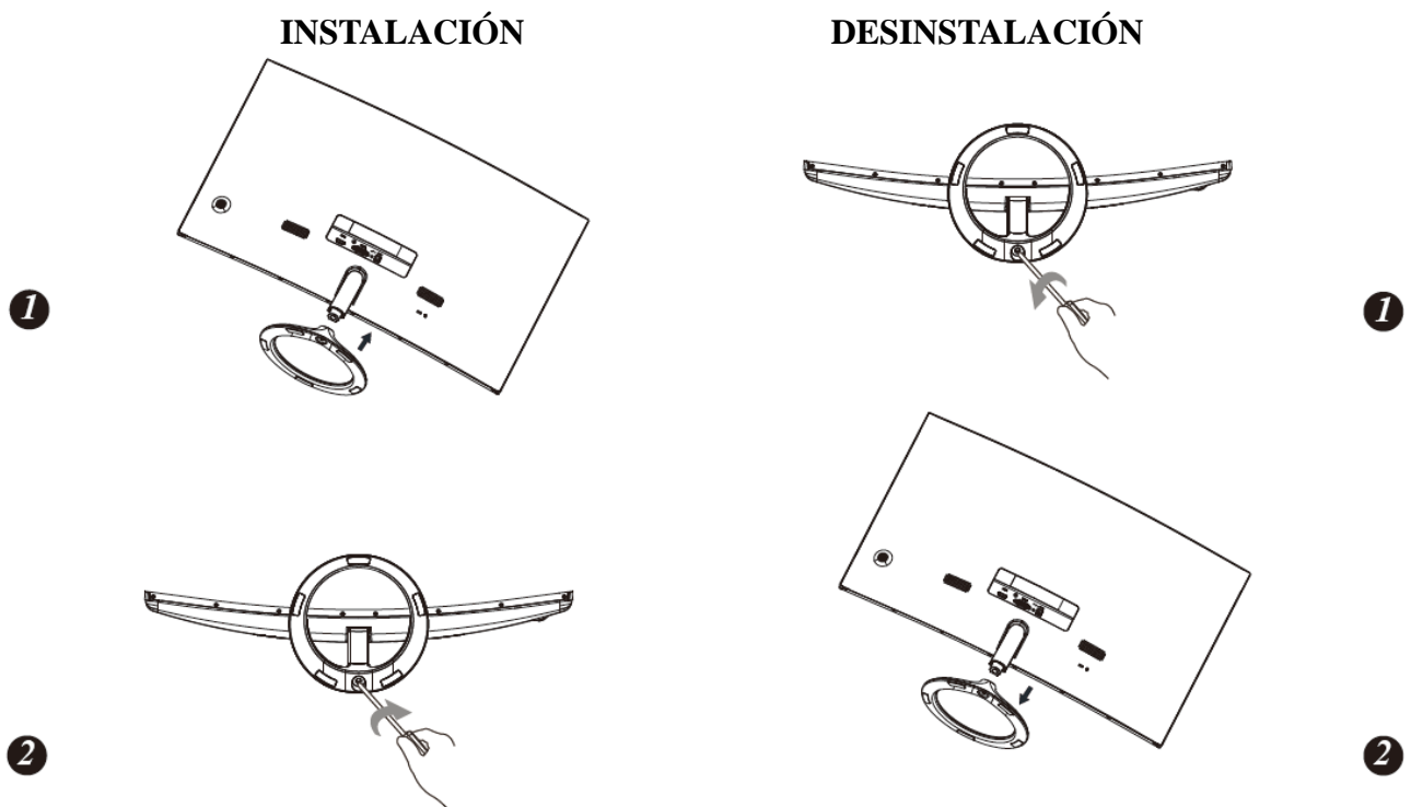
Figura 1. Instalar y desinstalar la base
