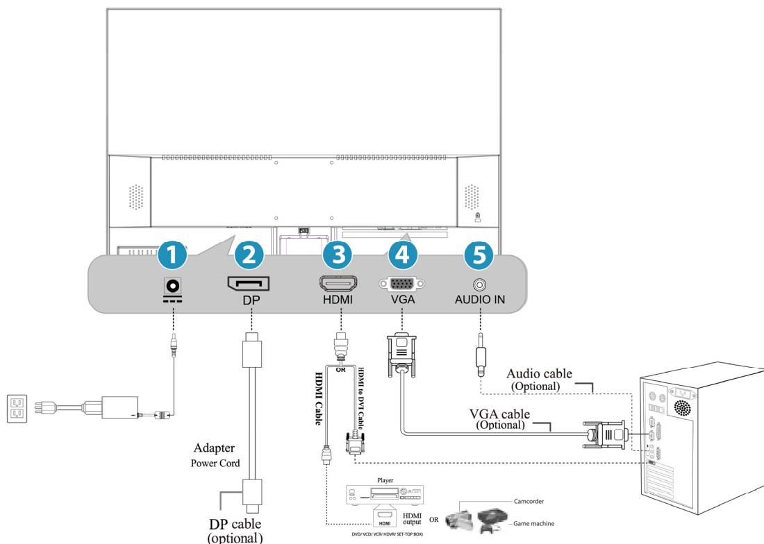
ABBILDUNG 2. ANSCHLISSEN AN EINEN PC
