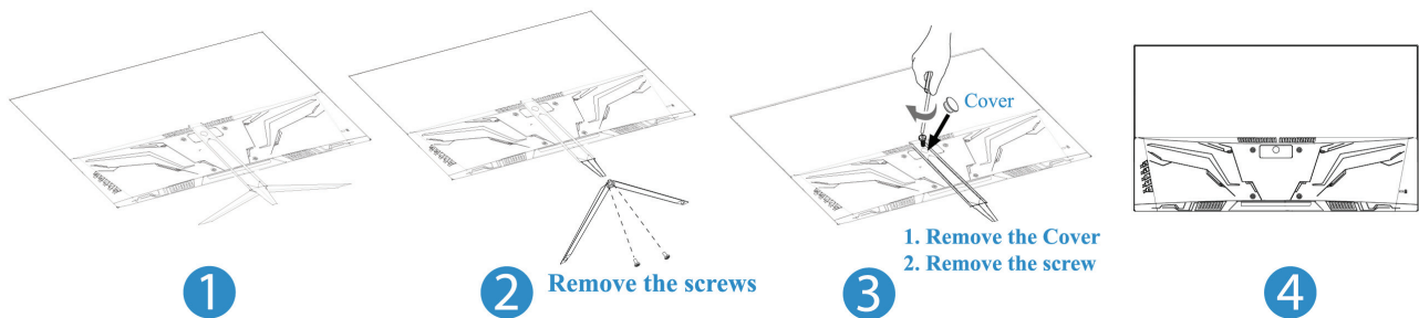
ABBILDUNG 1. INSTALLIEREN UND ENTFERNEN DES STÄNDERS
