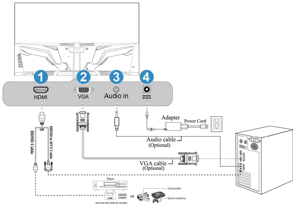
Figura 2. Branchement à un pc
