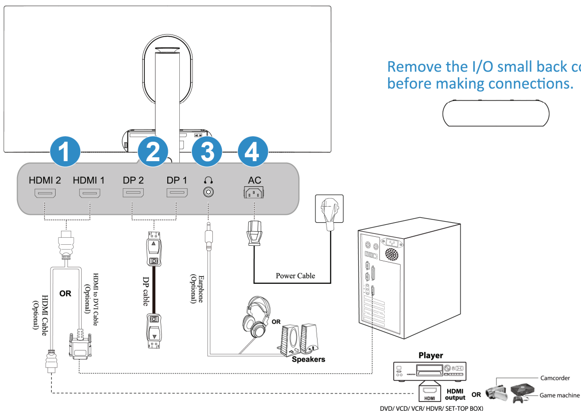
ABBILDUNG 2. ANSCHLISSEN AN EINEN PC
