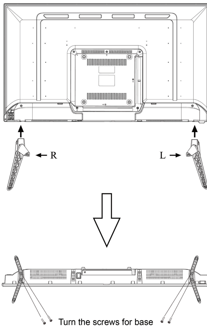
Figure.1. Installer et enlever l'embase
