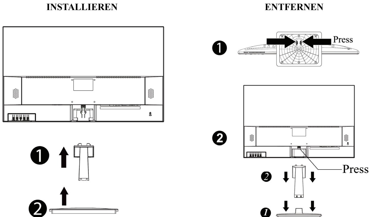
ABBILDUNG 1. INSTALLIEREN UND ENTFERNEN DES STÄNDERS
