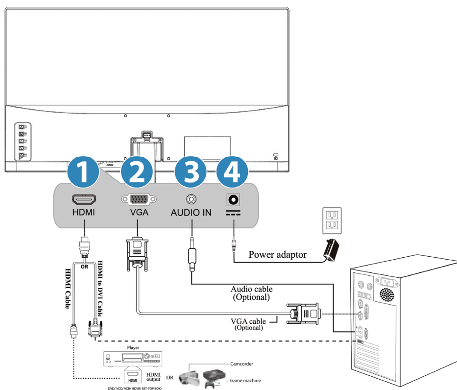
Figura 2. Branchement à un pc
