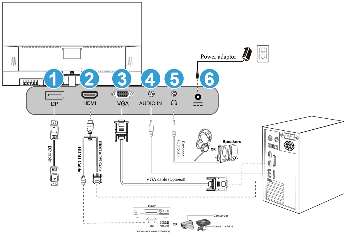
ABBILDUNG 2. ANSCHLISSEN AN EINEN PC
